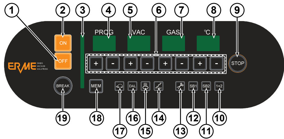
Fig. 14: Commande CP-E5
