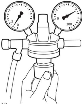
Abb. 12: Ventilarmatur
