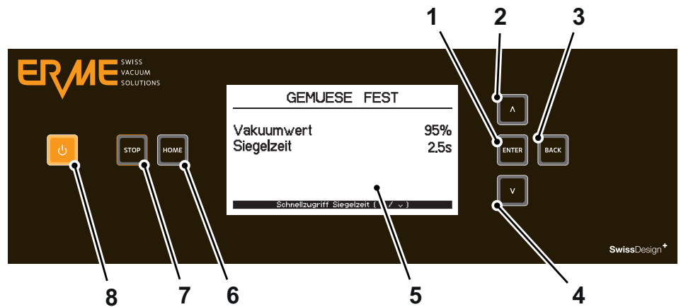
Imm. 5: Pannello di comando
