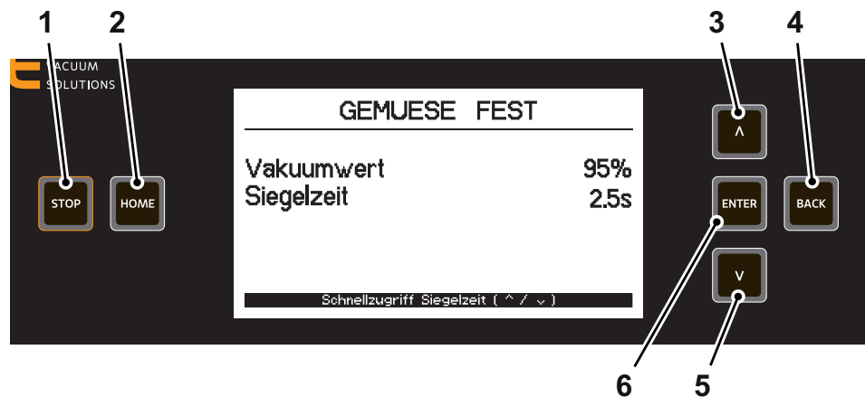
Imm. 13: Pannello di controllo della centralina CP-E3
