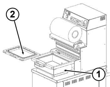
Imm. 28: Estrarre il cassetto con lo stampo
