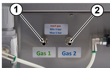
Imm. 21: Attacco per gas protettivo
