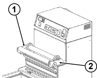
Imm. 24: Caricamento della bobina di pellicola
