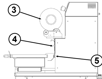
Imm. 25: Trascinamento della pellicola
