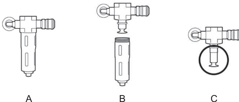
Fig. 15: Nettoyage du séparateur GreenVac
