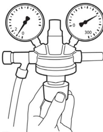
Fig. 12: Détendeur
