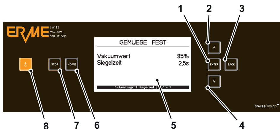
Fig. 5: Panneau de commande
