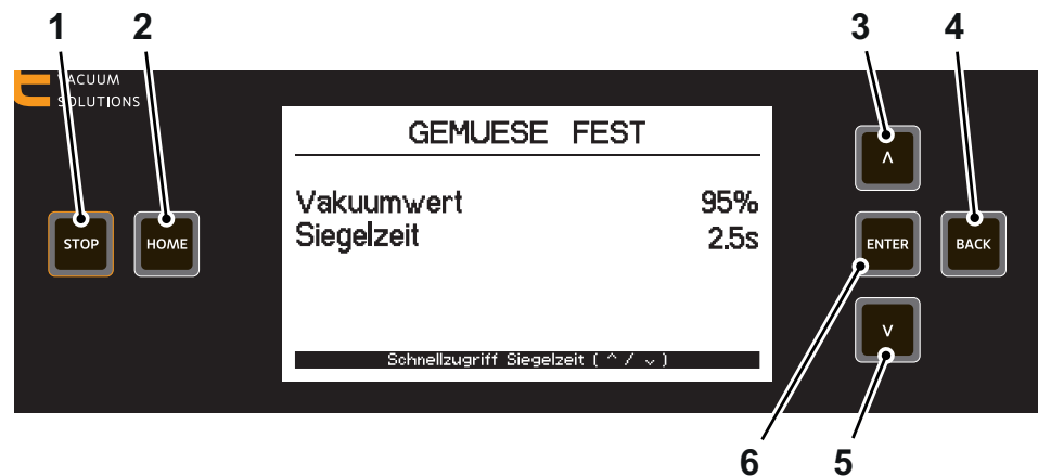
Fig. 13: Panneau de commande de la commande CP-E3
