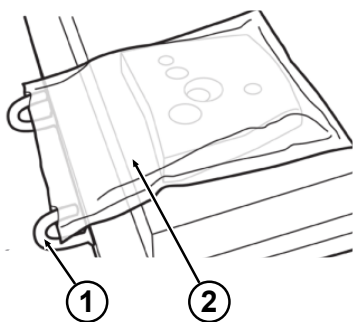
Fig. 13: Positionnement des buses (1) Buses (2) Sac d'emballage sous vide
