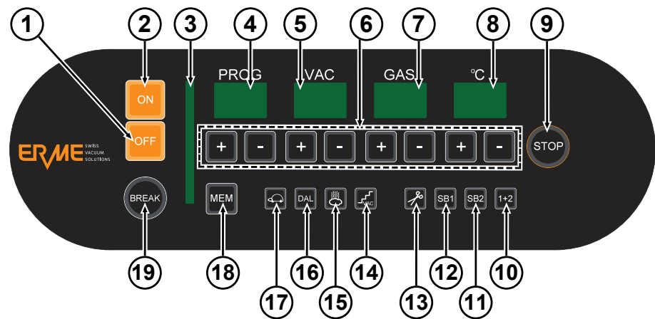
Fig. 5: Commande CP-E5
